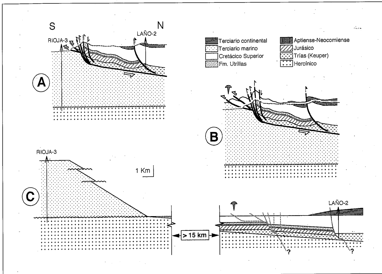
Fig. 4.— A: corte geológico actual; B: corte geológico considerando la roña erosionada; C: corte balanceado.
