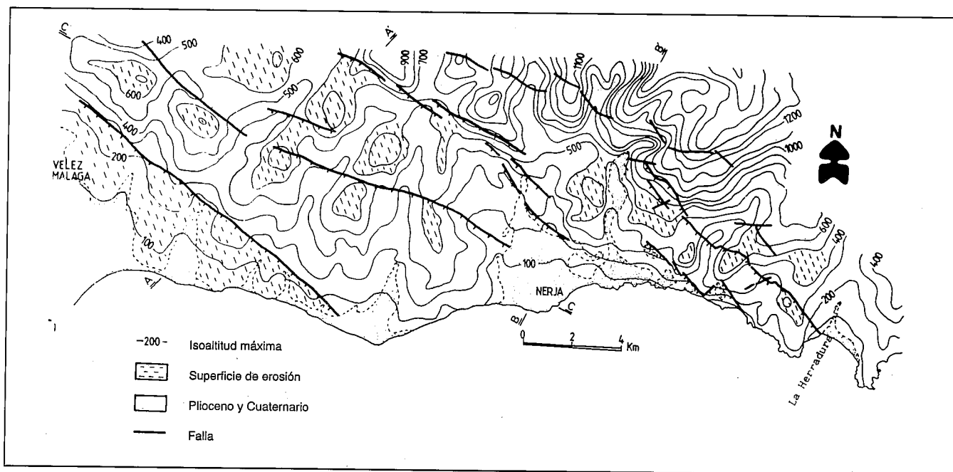
Fig. 2.—Mapa de envoltorio del relieve (tangencia superior), con restos de relieve aplanado y alineaciones tectónicas.
