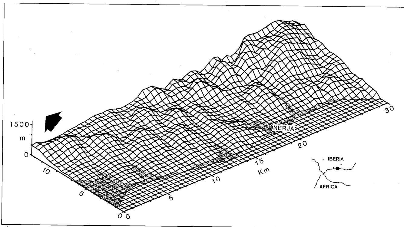
Fig. 1.—Bloque diagrama digitalizado del mapa de envoltorio del relieve (tangencia superior). Se indica, con punteado, la zona cubierta por depósitos plio-cuaternarios.
