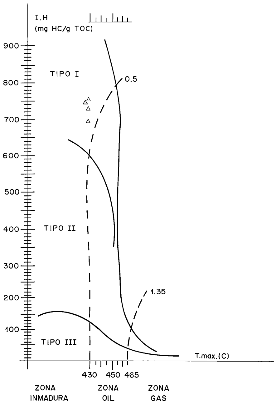
Fig. 2.—Situación de las muestras de la Tabla 1 en el diagrama HI-T máx.
