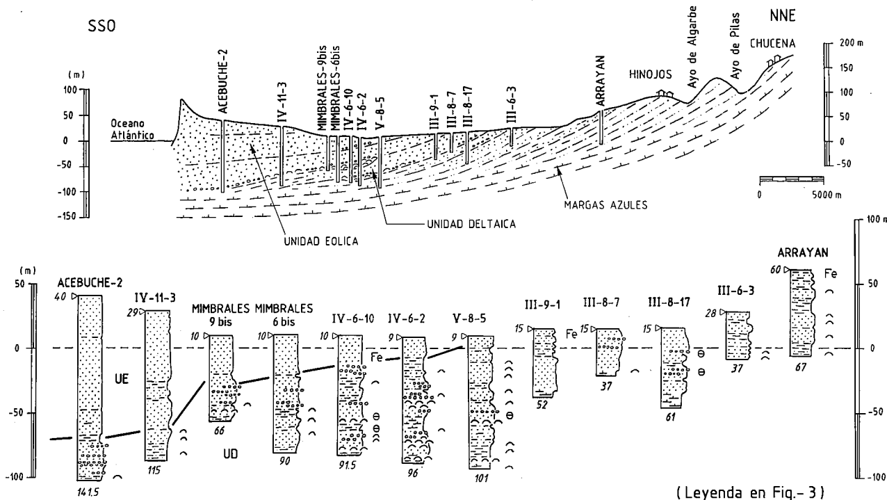
Figura 5.- Corte 3 y columnas litológicas en los depósitos plio-cuaternarios del Bajo Guadalquivir.
