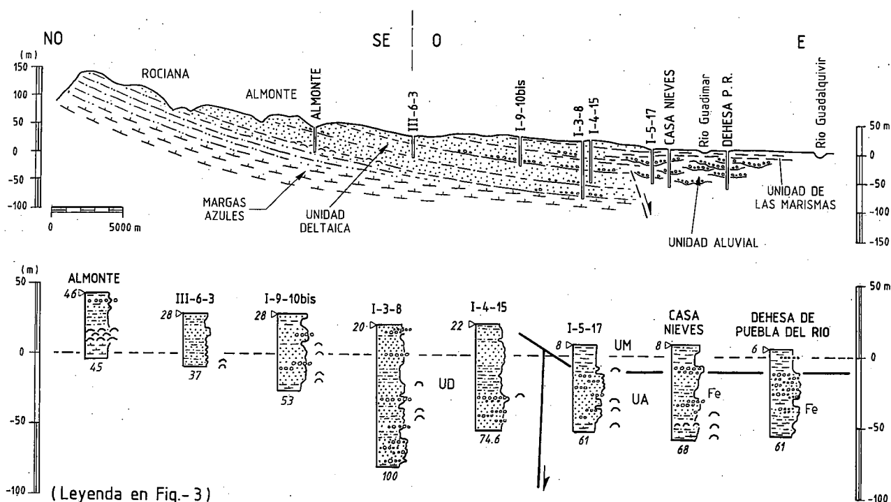
Figura 4.- Corte 2 y columnas litológicas en los depósitos plio-cuaternarios del Bajo Guadalquivir.
