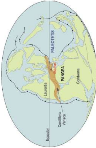
Fig 5. Paleogeografía durante el Carbonífero.
