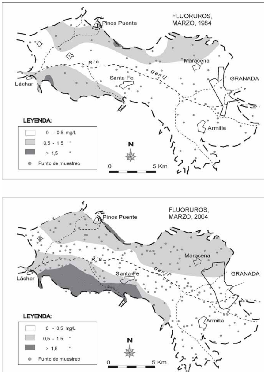
Fig. 3.- Mapas de isocontenidos en fluouros del acuífero de la Vega de Granada para marzo de 1984 y 2004.
