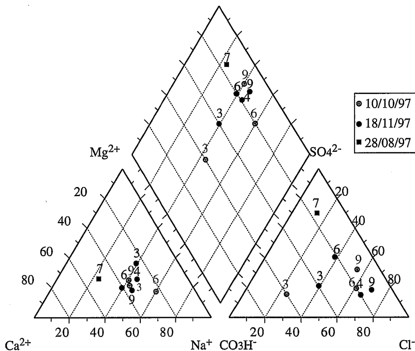
Fig. 2- Diagrama de Piper de las muestras analizadas.
