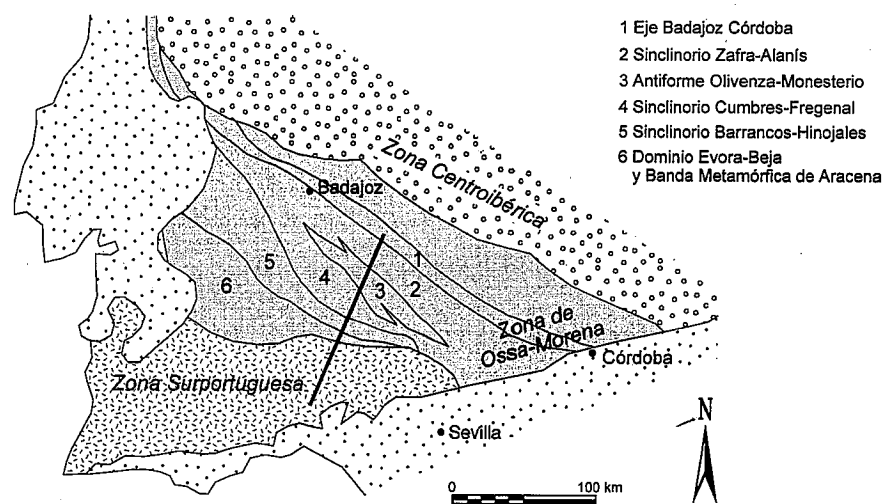
Figura 1. Situación geográfica y geológica de la zona estudiada y localización del perfil.
