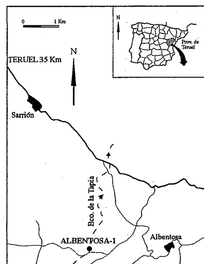
Fig. 1.- Localización geográfica del afloramiento Albentosa -1.
