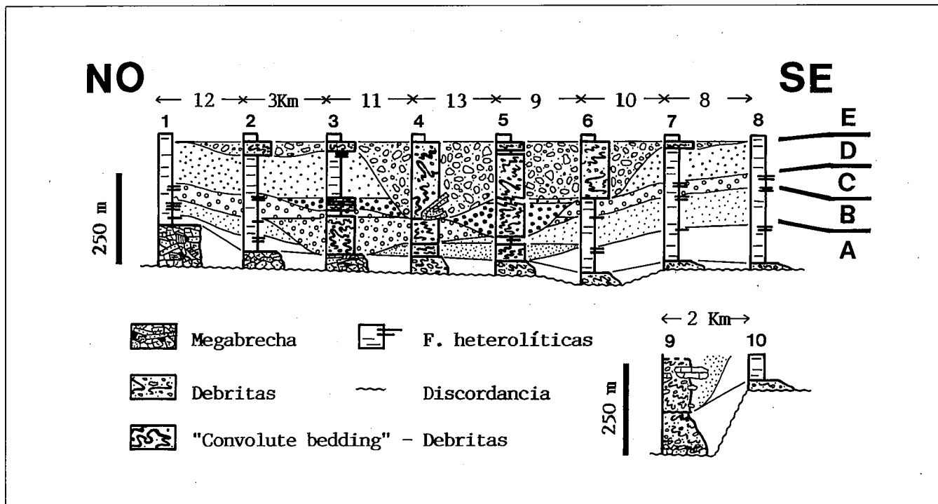
Fig 2.— Cambios laterales del Nivel de Fuentes e individualización de cinco subunidades. Localidades: 1: A. Pedroso, 2: A. Fuentes, 3: Río Uso, 4: Río Frío, 5: Río Fresnedoso, 6: Río Estenilla, 7: Río Estena, 8: A. Bohonal, 9: Casas del Membrillar, 10: E Casa del Membrillar.
